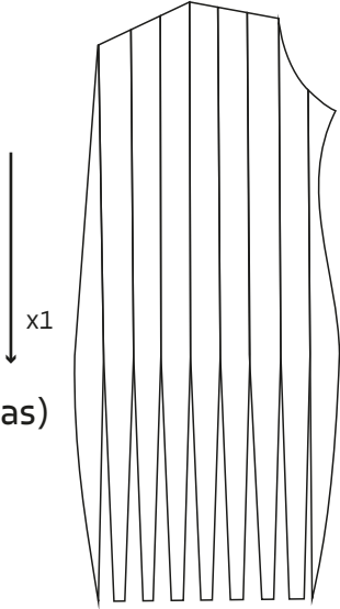
Pierna delantera B (9 piezas) T.B Sastrero Talle: M Pantalón conjunto Art. nº0-202
